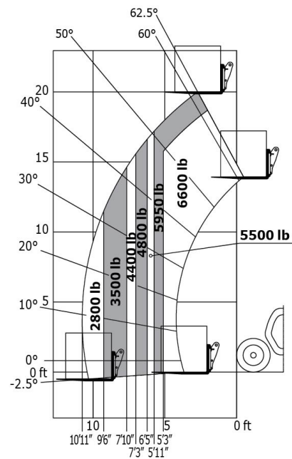
Rough terrain load chart (EN 1459 B) Metric Rough terrain load chart (EN 1459 B) Imperial
