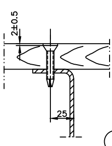
SECTION F-F 1 : 2
