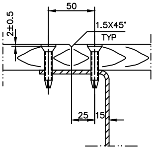
SECTION E-E 1 : 2
